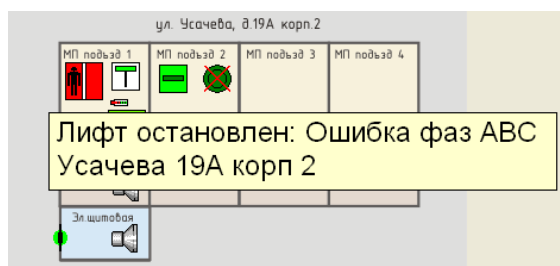
Рисунок 25 - Срабатывание устройства контроля следования фаз
