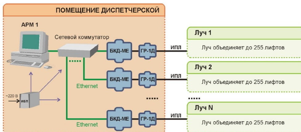
Рисунок 12 - Вариант построения многолучевой однопользовательской системы СЛДКС-1
