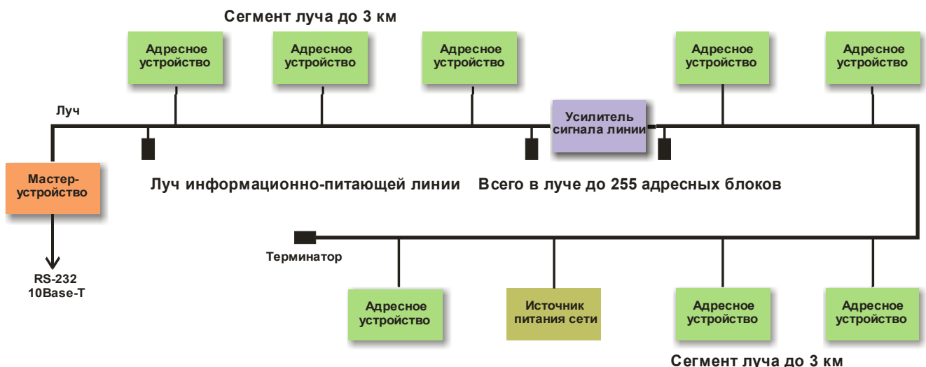
Рисунок 1 - Типовая схема подключения устройств интерфейса ИПЛ
