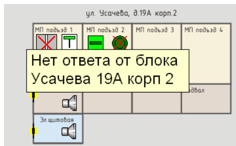
Рисунок 40 - Нет связи с адресным блоком
