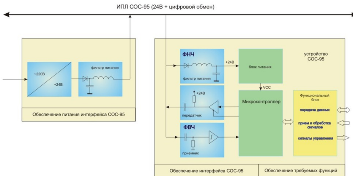
Рисунок 3 - Типовая блок-схема устройства с интерфейсом СОС-95-FAST
