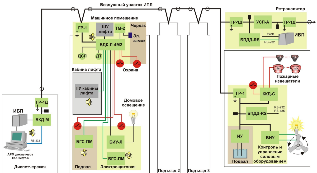
Рисунок 7 - Схема типового оснащения жилого дома
