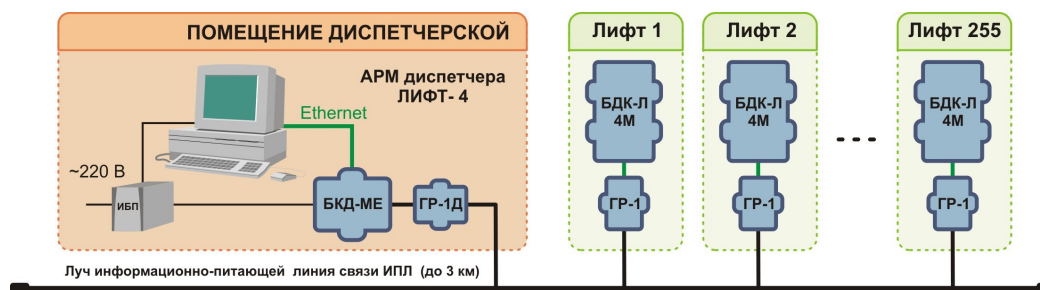
Рисунок 11 - Однопользовательский однолучевой вариант СЛДКС-1 с интерфейсом Ethernet
