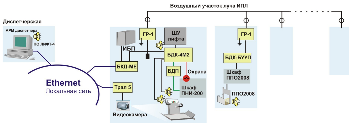
Рисунок 20 - Диспетчеризация платформ подъемных для инвалидов
