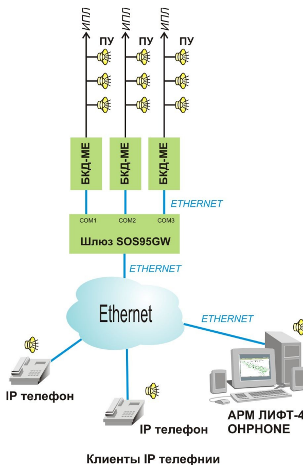
Рисунок 19 - Структура IP телефонии
