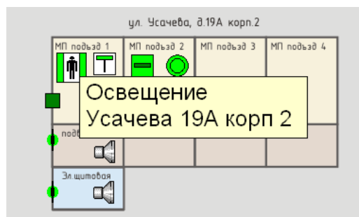
Рисунок 31 - Включение группы освещения
