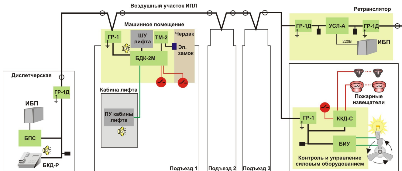
Рисунок 8 - Структурная схема СЛДКС-1 без компьютера
