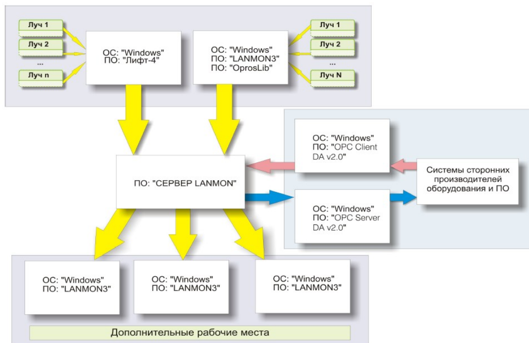
Рисунок 21 - Программное обеспечение СЛДКС-1
